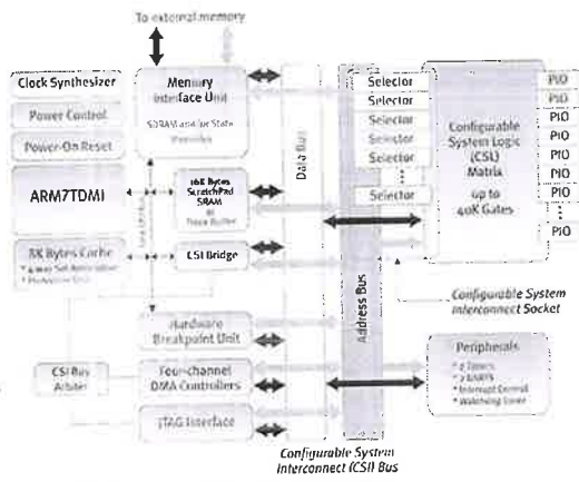
Triscend's A7 CSoC
